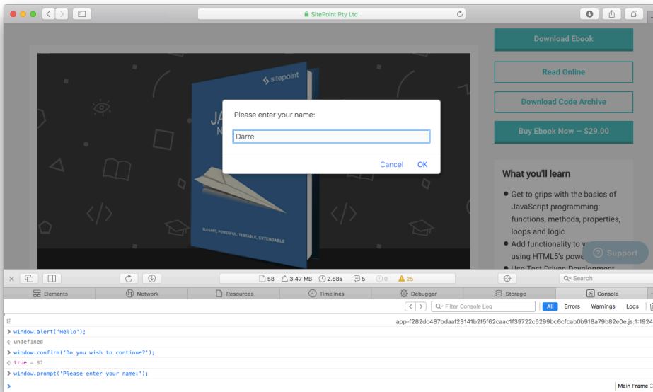
9-3. Prompt dialog
