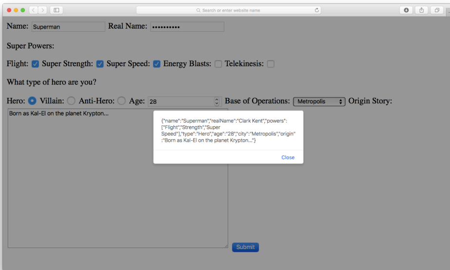
8-5. Hero JSON
