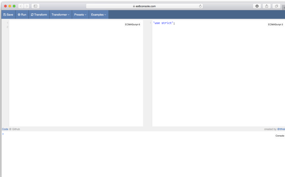
1-3. ES6 Console
