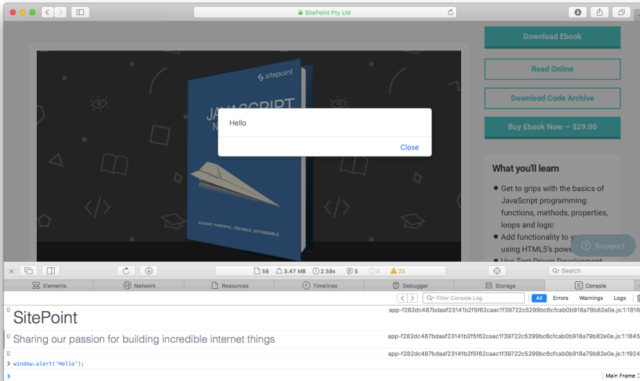
9-1. Alert dialog
